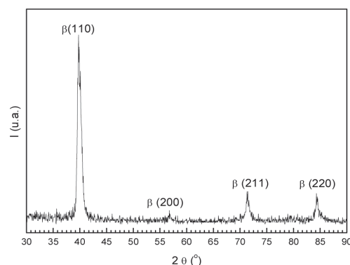
Figura 1- Difratograma de raios X da liga Ti-12Mo-3Nb tratada a 950°C/1h.
