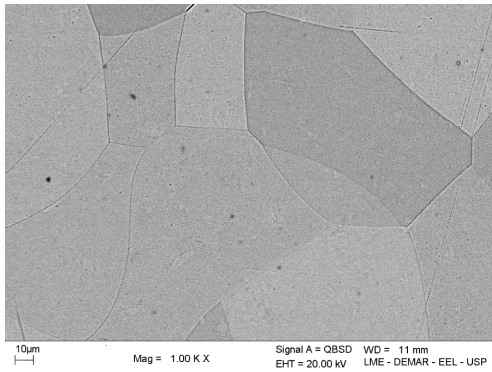
Figure 2- Micrografia da liga Ti-12Mo-3Nb tratada a 950°C/1h.
